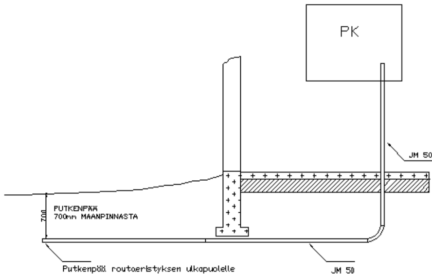
Kuva 1. Liittymiskaapelin putkitus,
