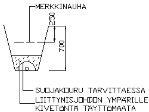
Kuva 2. Liittymisoja
