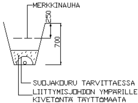
Kuva 2. Liittymisoja
