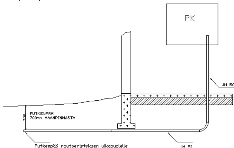
Kuva 1. Liittymiskaapelin putkitus,
